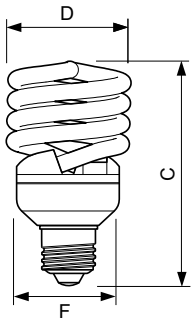
Twister 23W/770 E27 220-240V 50Hz
