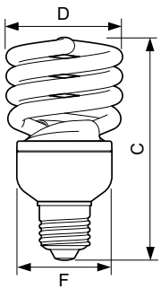
Twister 23W/770 E27 220-240V 50Hz
