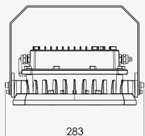
Vista em Elevação Elevated View / Vista Elevada
