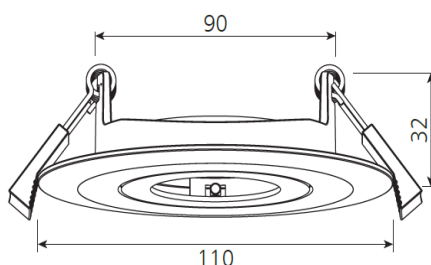
Tilt Trim Ø95
