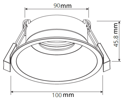
Deep Trim Ø90
