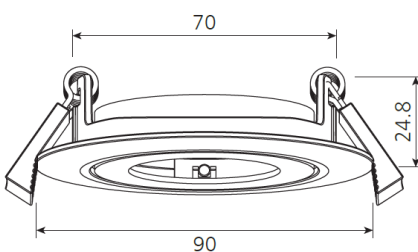
Tilt Trim Ø80
