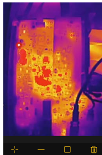
Alarma de área de exceso de temperatura
