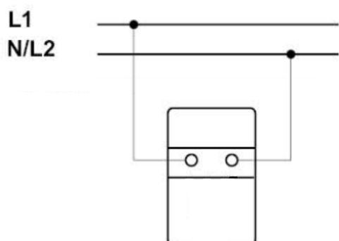
Diagrama de instalación
